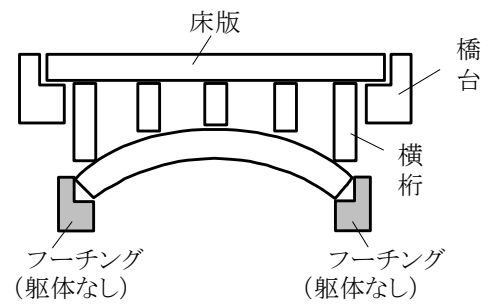
(3) アーチ橋
