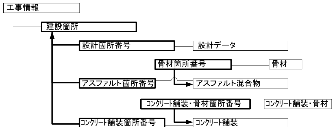
舗装情報関連概念図(建設時)
