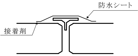
II-A型(頂版)
