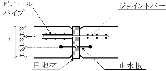
III型(底版)
