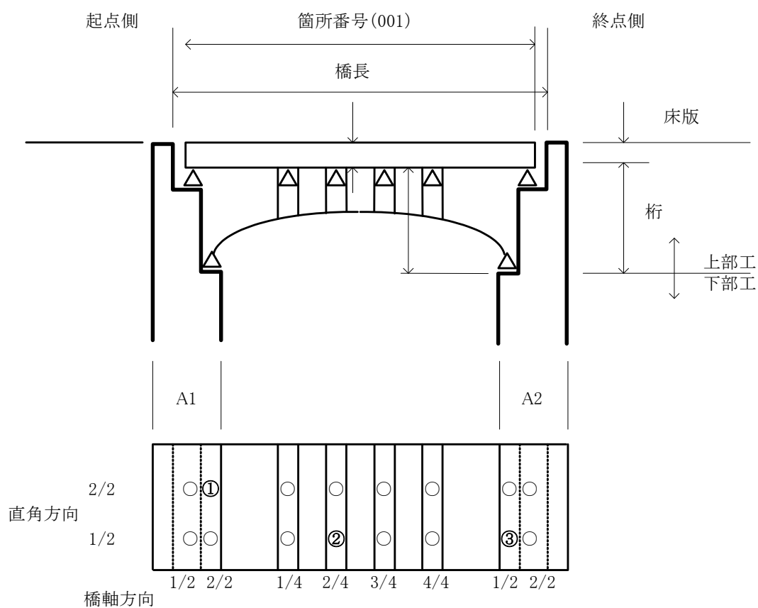
(h) アーチ橋の垂直材に支承がある場合
