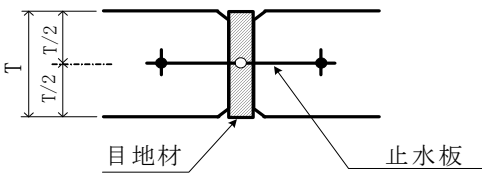
II-B型(側壁)
