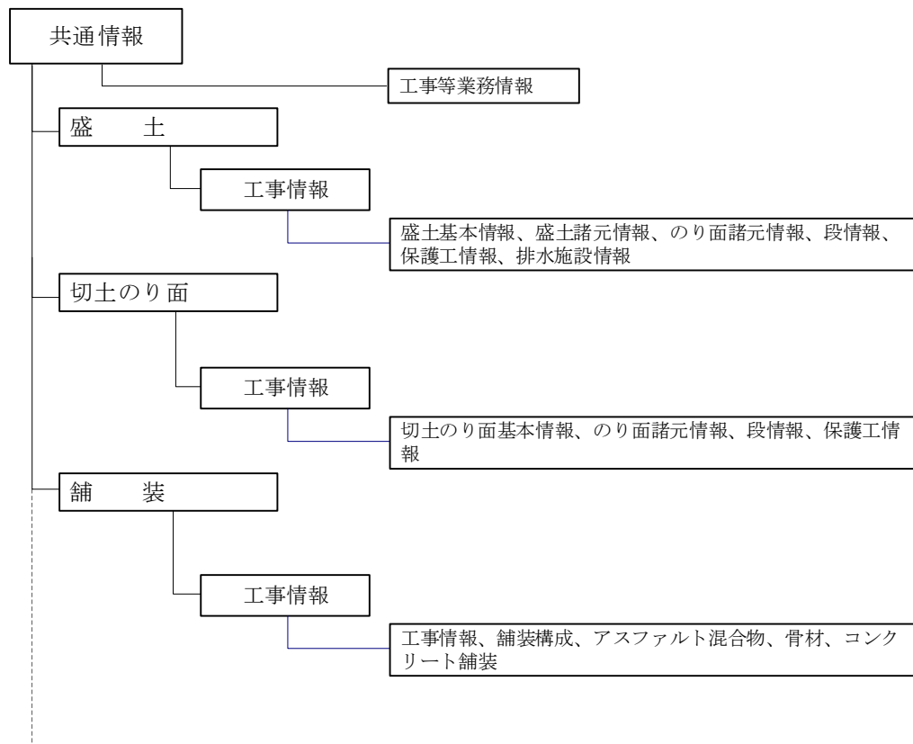
図 3-2 工事記録情報の構成概念図
