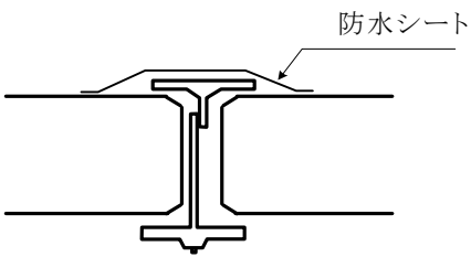
II-B型(側壁)
